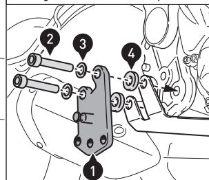
Montage mit SW-MOTECH Bugspoiler Mounting with SW-MOTECH Front Spoiler
